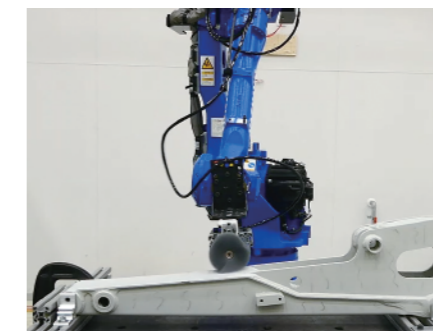
研磨ロボット設備
